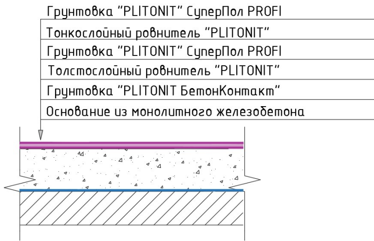
Сечение пирога пола.
